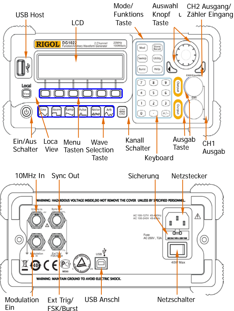
Bild 1 Vorder- und Rückseite Übersicht
